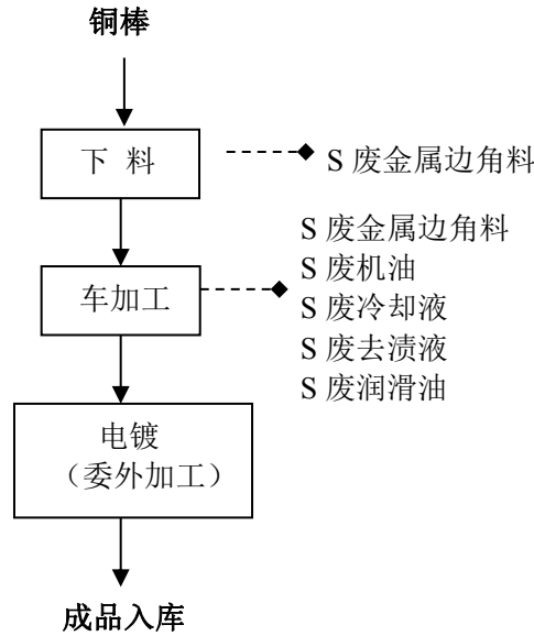
图 6-1 本项目电子接插件加工工艺流程及产污环节图
