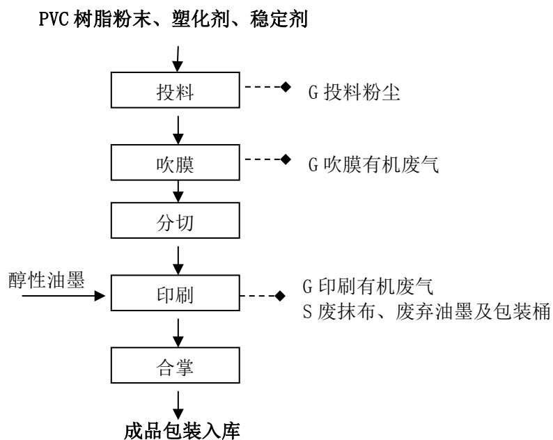
图 2.2-1 本项目塑料制品生产生产工艺流程及产污环节框图
