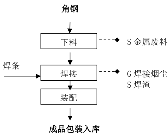
图 2.2-2 本项目五金机械生产生产工艺流程及产污环节框图
