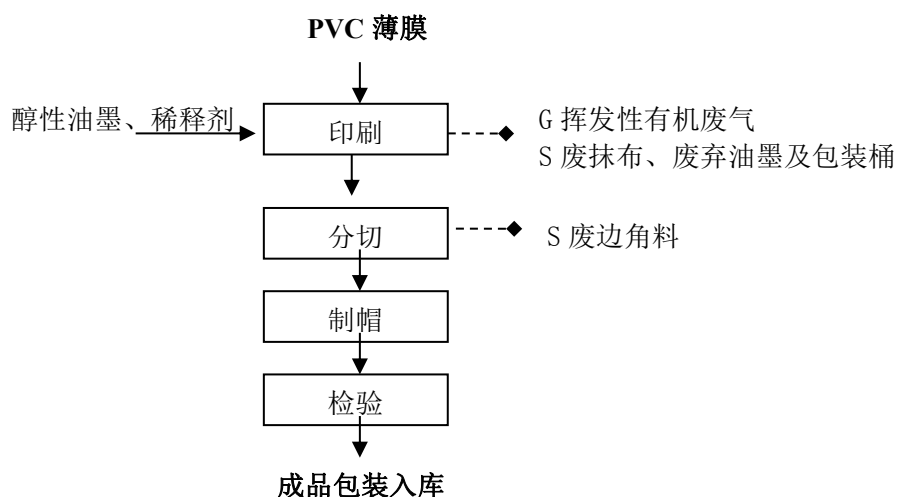
图 2.2-2 本项目塑料瓶套生产工艺流程及产污环节框图
