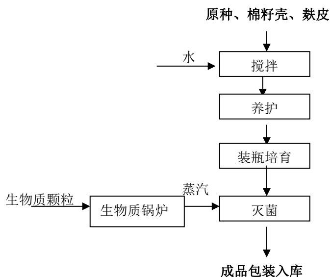
图 2.2-1 本项目食用菌菌种培育工艺流程及产污环节框图
