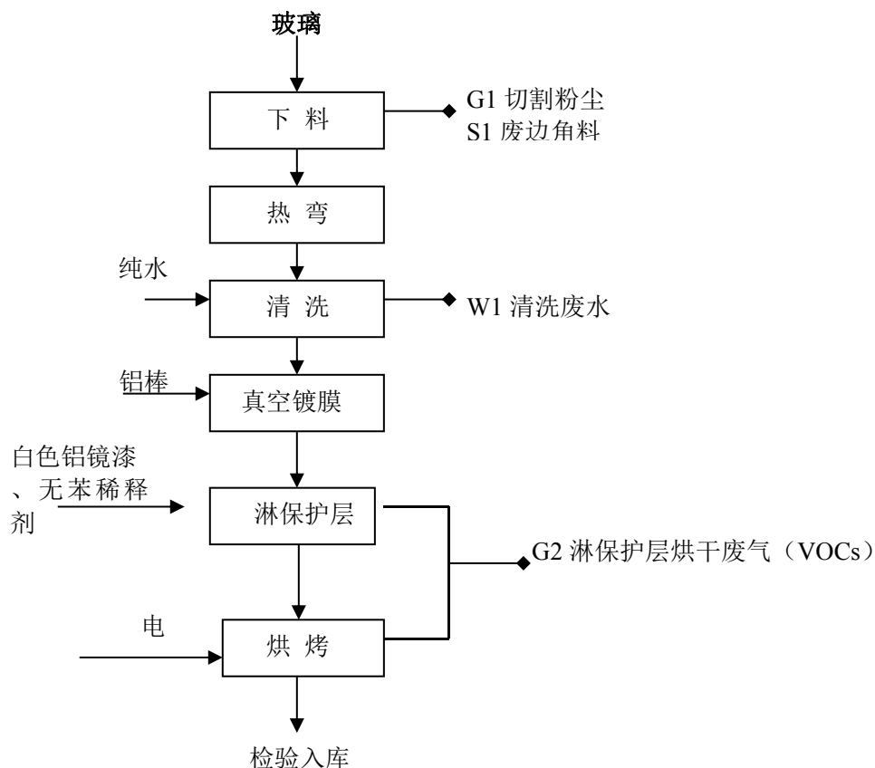
图 2.2-1 本项目汽车后视镜镜片生产工艺流程及产污环节图 工艺说明：
