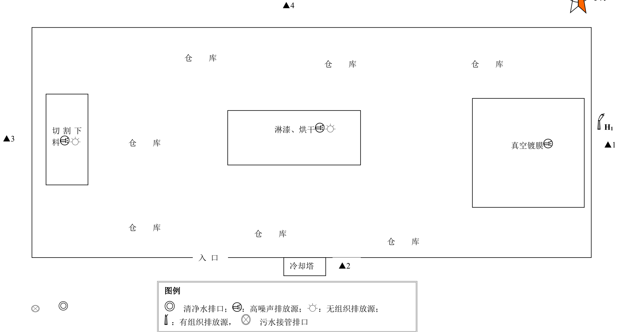
附图2 本项目平面布置图(附噪声监测点位)
