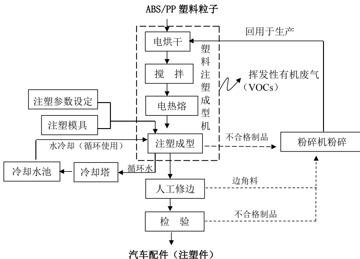
图 2.2-1 本项目生产工艺流程及产污环节图
