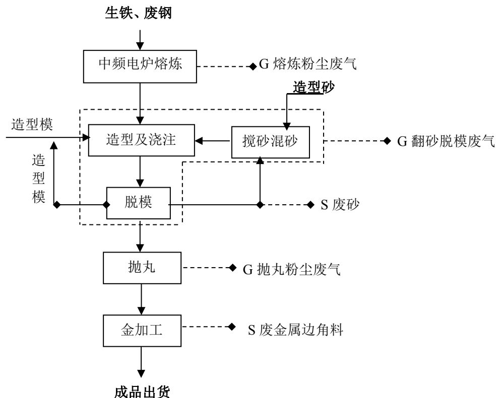
图 2.2-1 本项目锅炉配件生产工艺流程及产污环节框图
