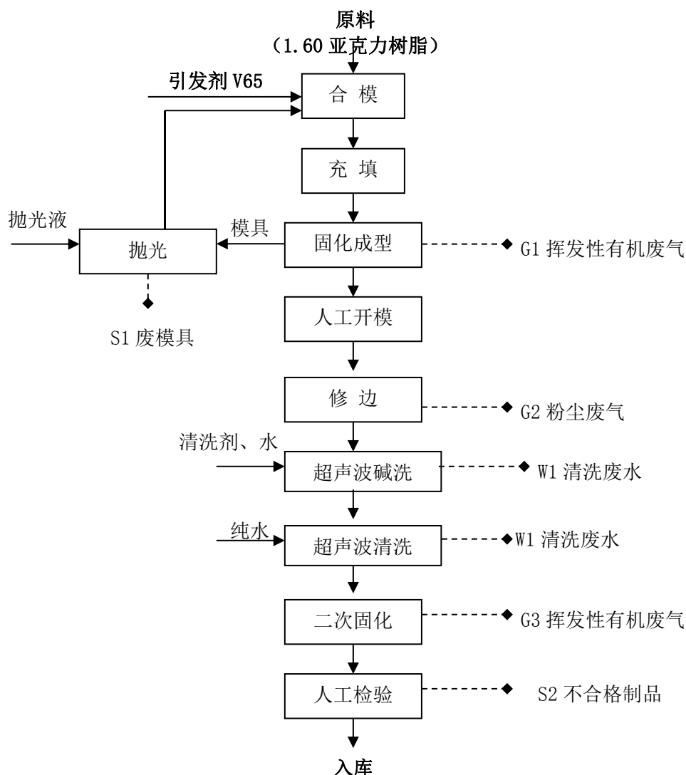
图 2.2-1 光学镜片生产工艺流程及产污环节框图
