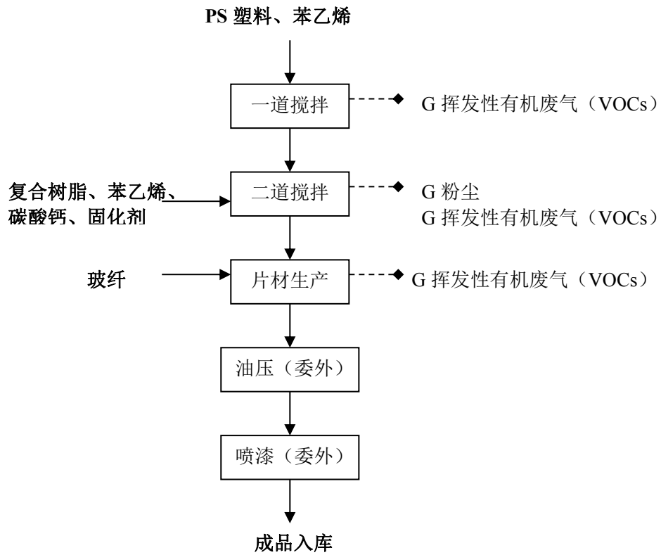
图 2.2-1 SMC 片材生产工艺流程及产污环节图
