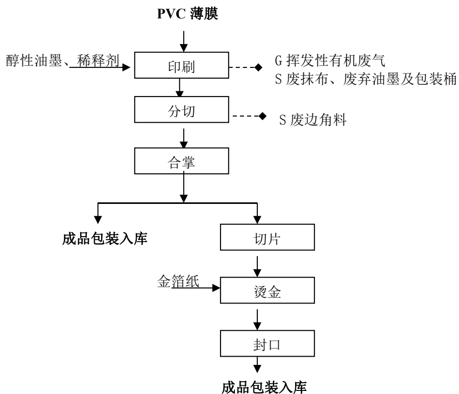
图 2.2-1 本项目塑料薄膜制品生产工艺流程及产污环节框图
