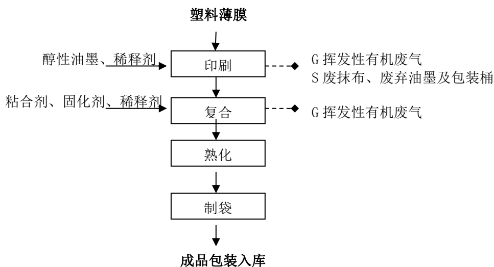
图 2.2-1 本项目包装袋生产工艺流程及产污环节框图
