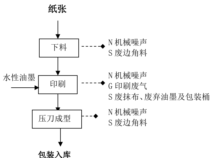
图 2.2-1 本项目纸包装制品生产工艺流程及产污环节图 生产工艺流程简述如下:
