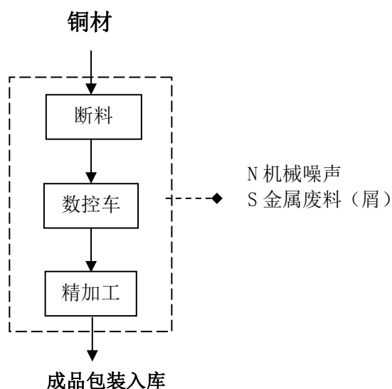
图 2.2-1 本项目五金工具生产工艺流程及产污环节图
