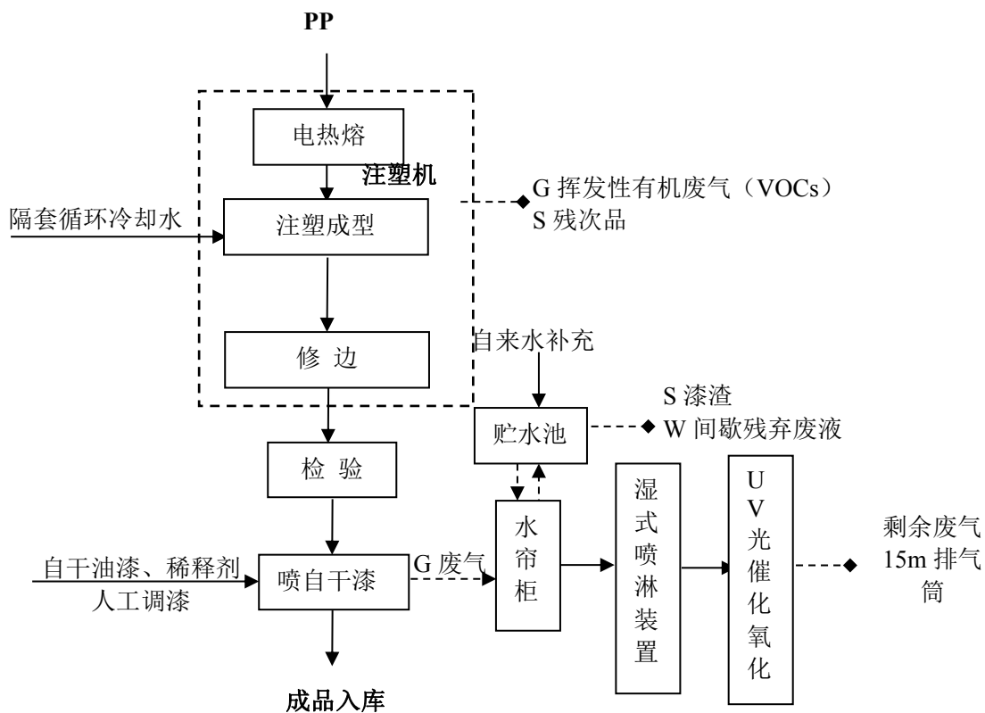
图 2.2-1 本项目挡泥板、门框生产工艺流程及产污环节图
