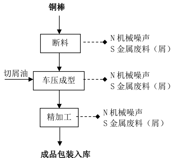
图 2.2-1 本项目电子接插件生产工艺流程及产污环节图
