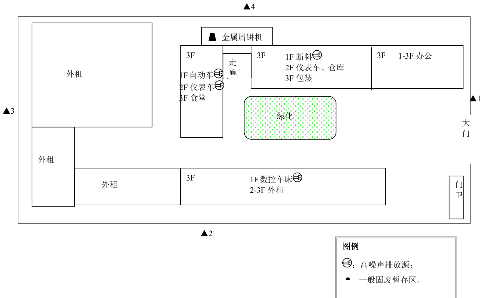
附图2 本项目厂区平面布置图（附噪声监测点）
