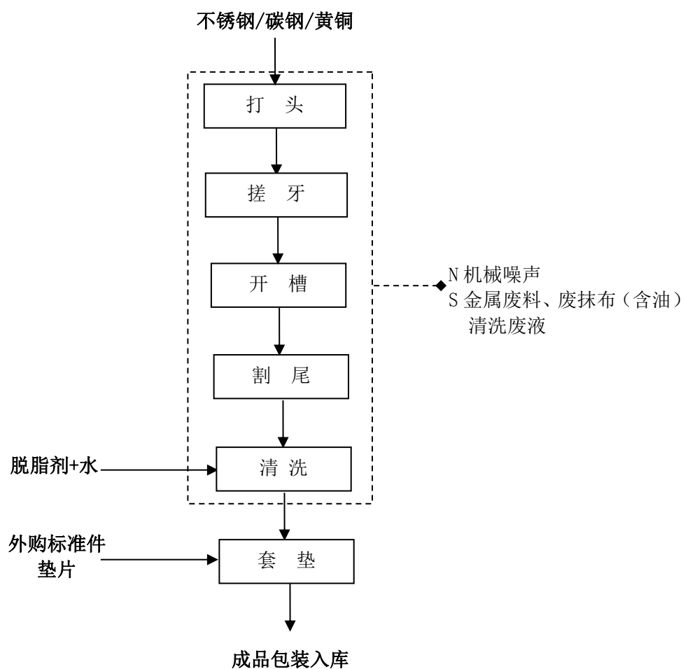
图 2.2-1 本项目生产工艺流程及产污环节框图
