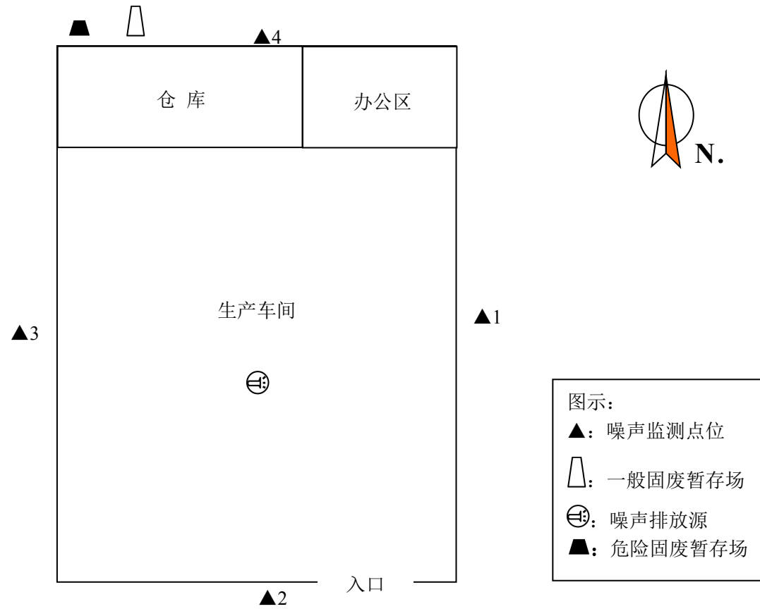
附图2 本项目厂区平面布置图（附噪声监测点位）
