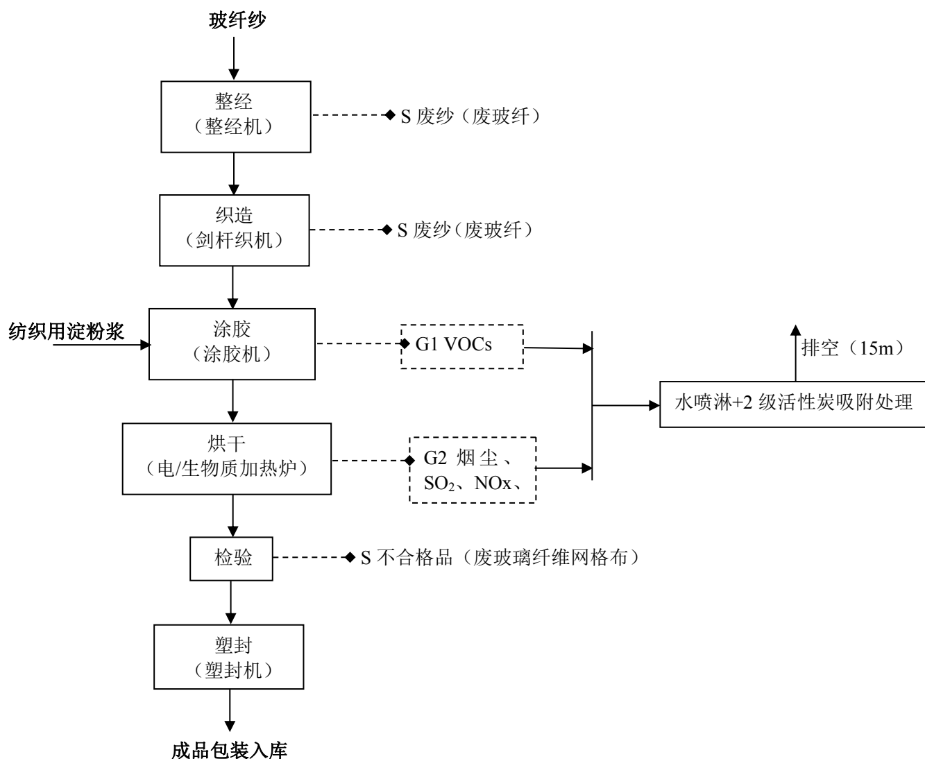
图 2.2-1 本项目生产工艺流程及产污环节图
