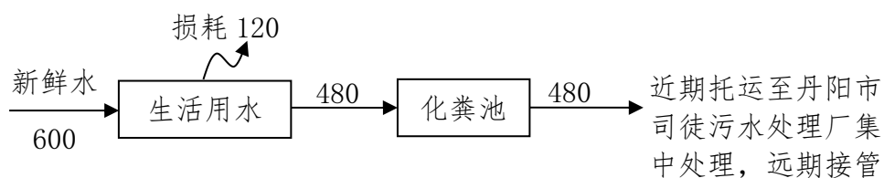
图 2.2-2 本项目用水排水平衡图 (t/a)
