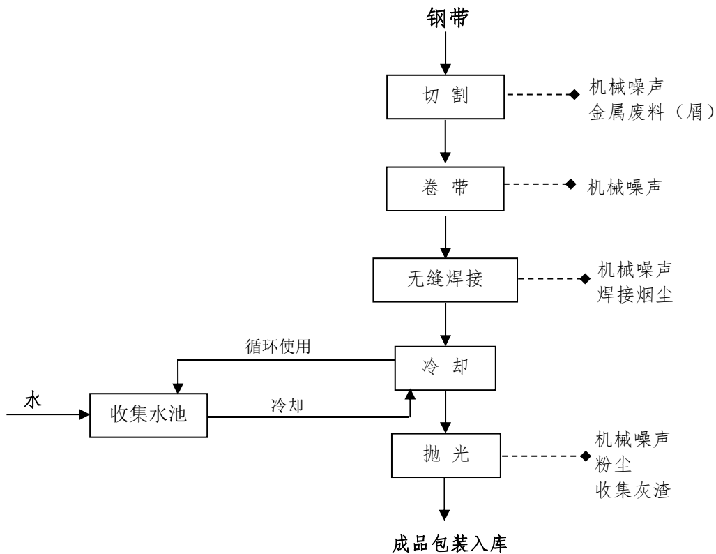
图 2.2-1 本项目生产工艺流程及产污环节图
