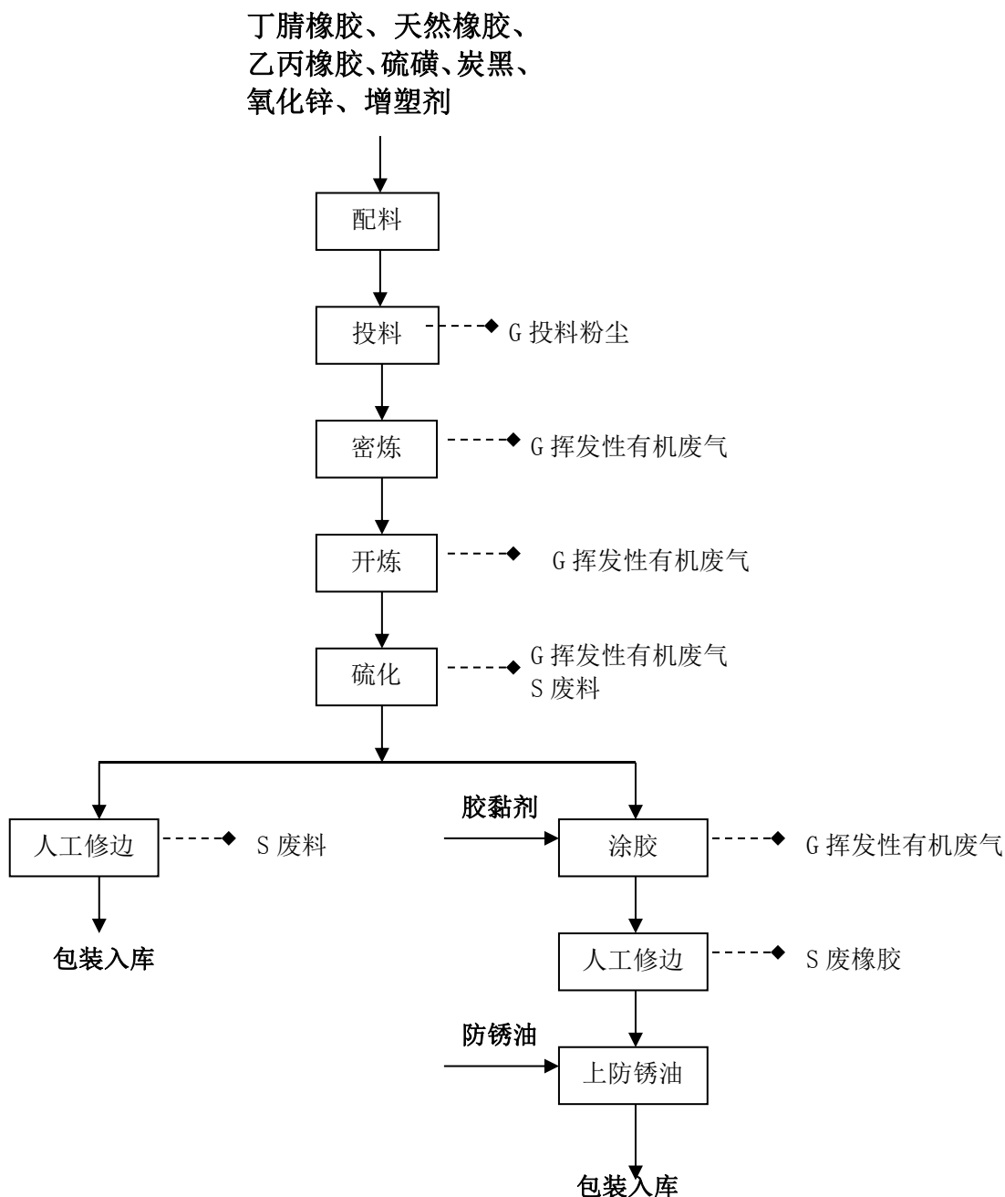
图 2.2-1 本项目橡塑制品生产工艺流程及产污环节图
