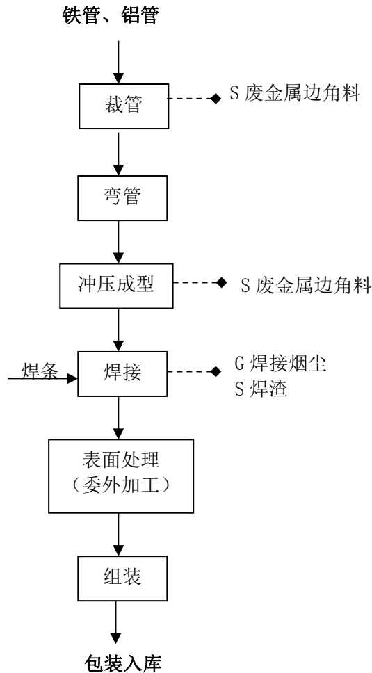
图 1 手动轮椅、电动轮椅、便器椅、助行器生产工艺流程及产污环节框图
