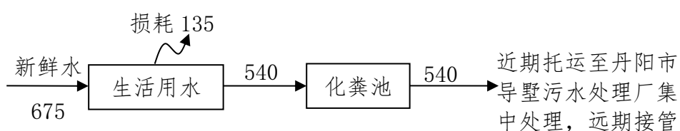
图 2.2-2 本项目用水排水平衡图 (t/a)
