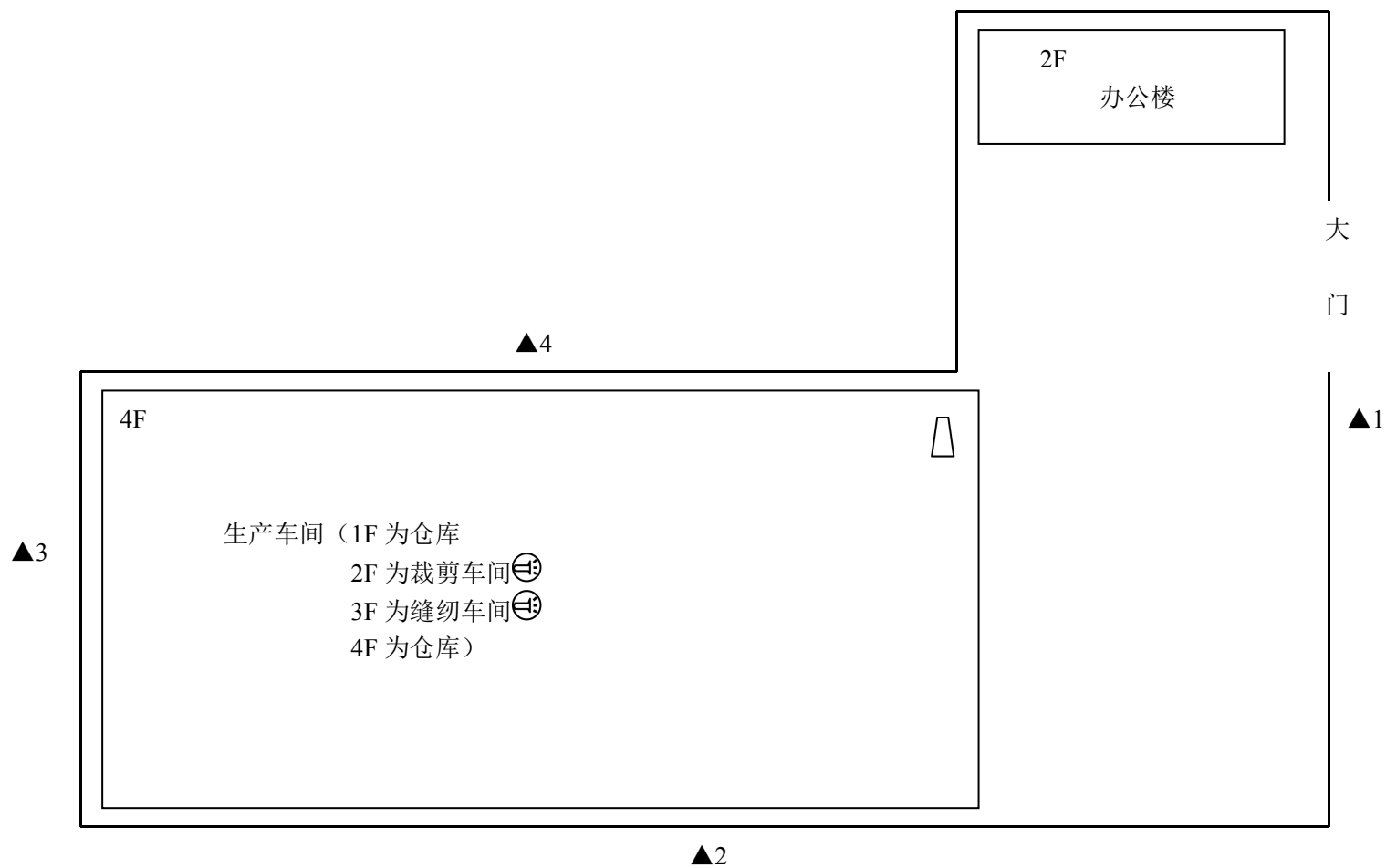
附图2 本项目厂区平面布置图（附噪声监测点位）
