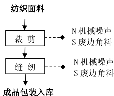
图 2.2-1 本项目旅游用品生产工艺流程及产污环节框图
