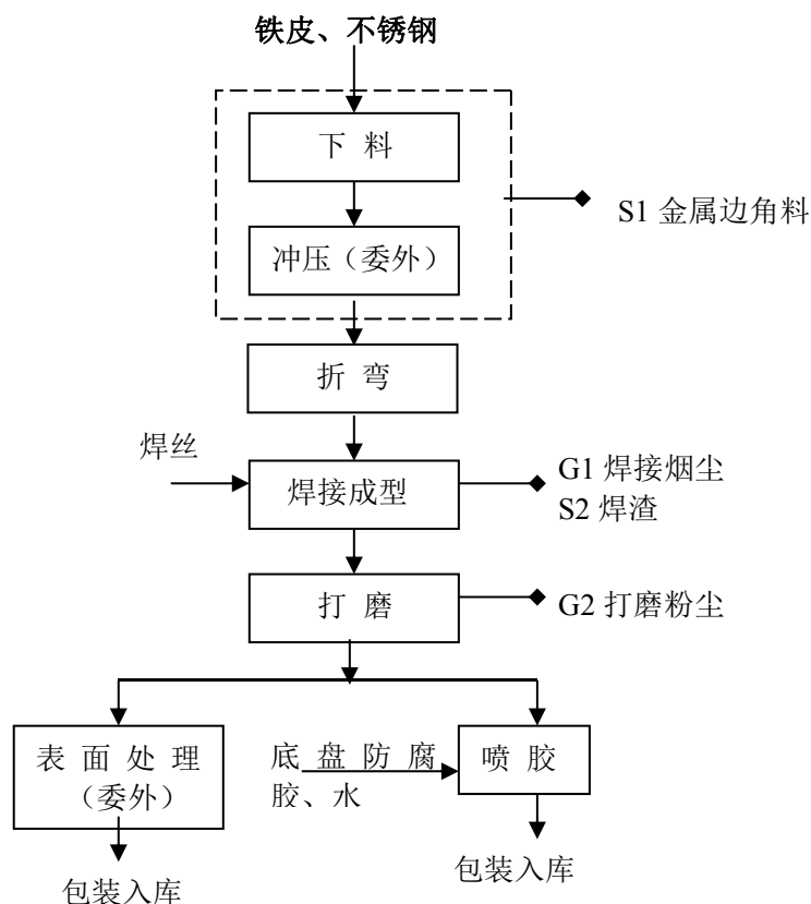
图 2.2-1 本项目汽车钣金件生产工艺流程及产污环节图
