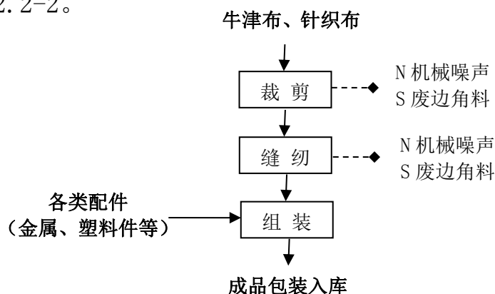
图 2.2-1 本项目帐篷、防护罩生产工艺流程及产污环节框图
