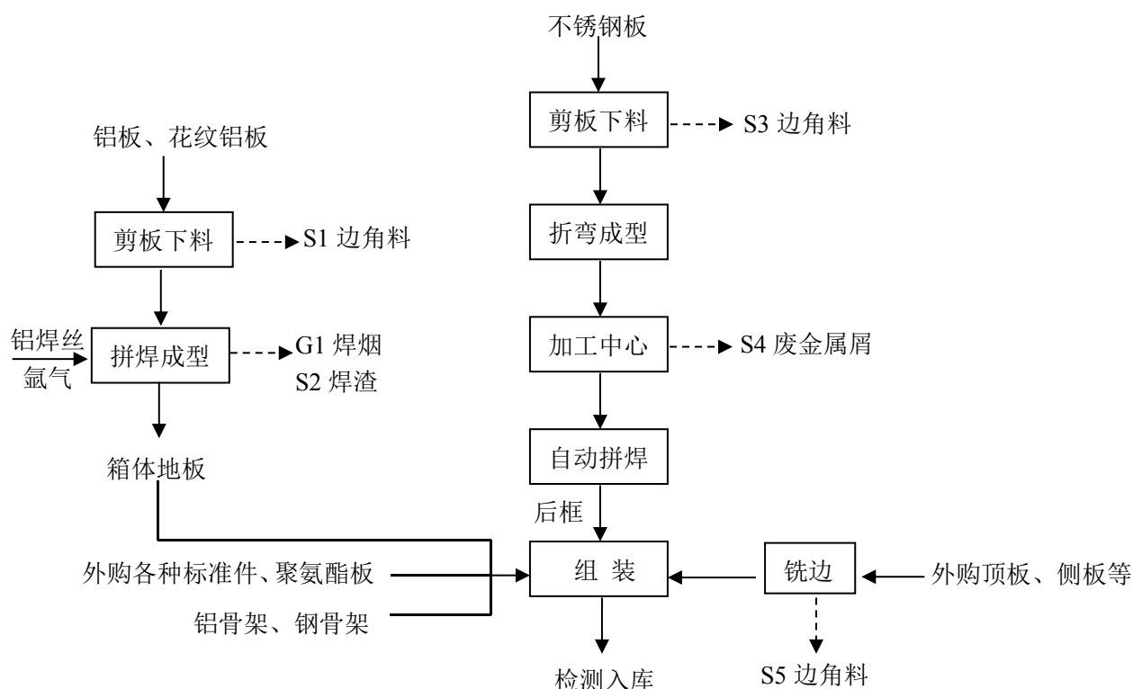
图 6-1 冷藏车箱体工艺流程图
