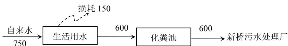
图 6-2 全厂用排水平衡图（t/a）
