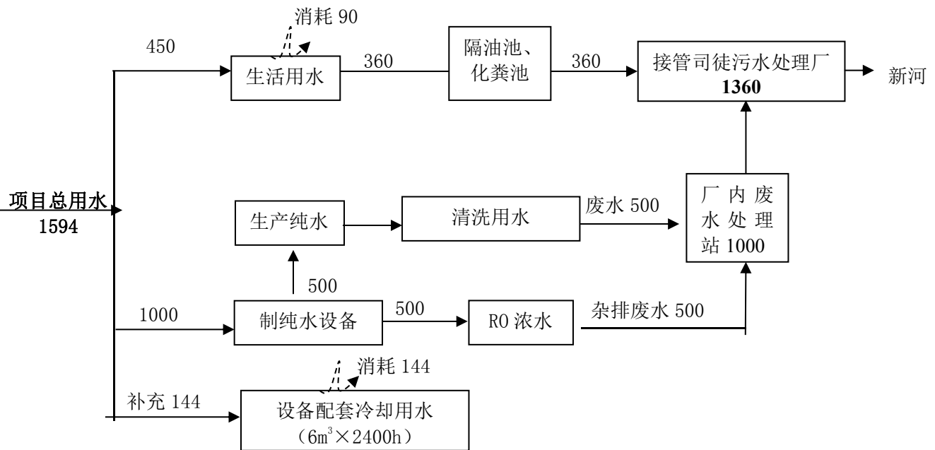
图 2 本项目水量平衡图 (单位: t/a)
