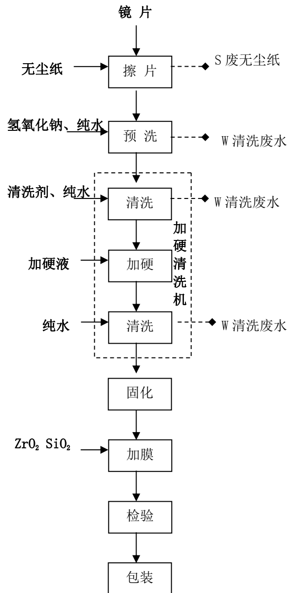
图 1 树脂镜片加硬加膜生产工艺流程及产污环节框图
