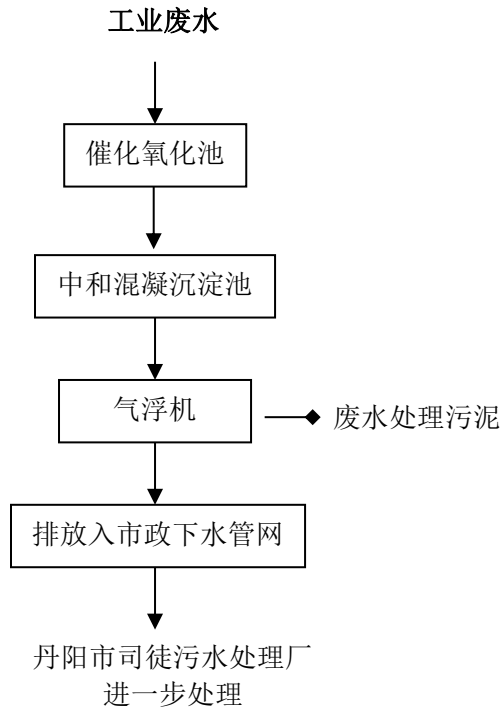
图3 工业废水预处理工艺流程图
