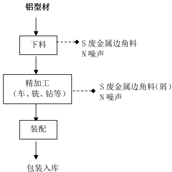
图 1 医疗器械配件生产工艺流程及产污环节框图
