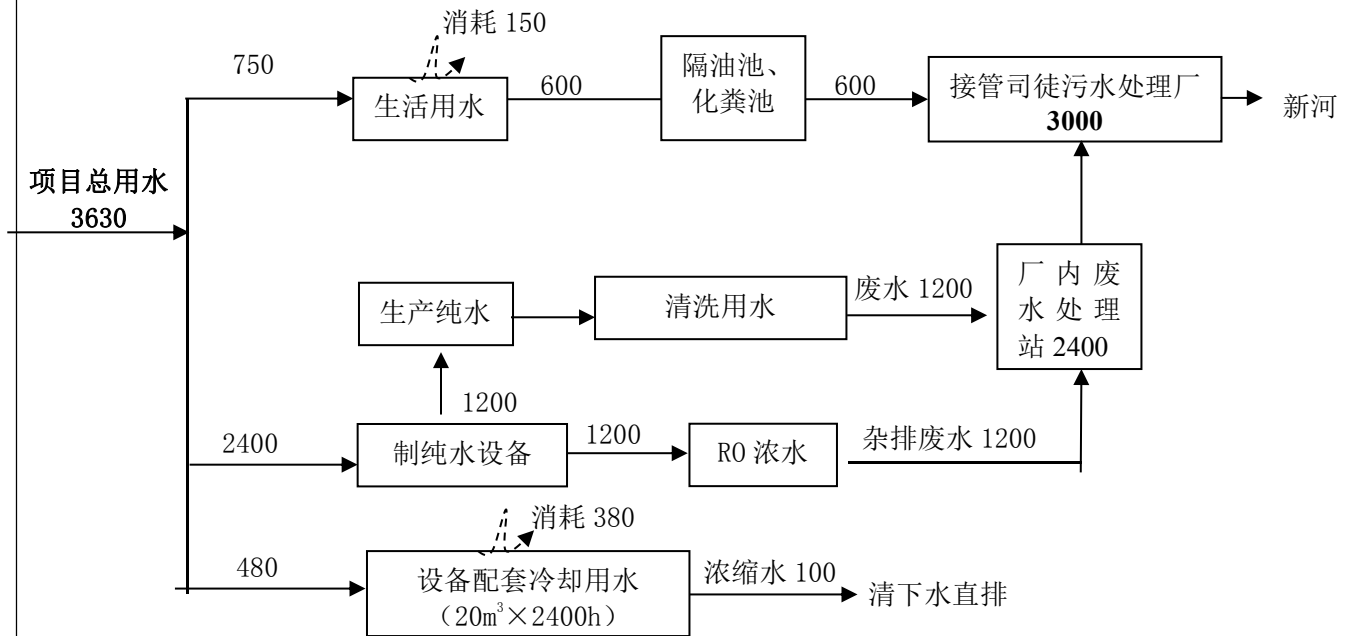
图 2 本项目水量平衡图（单位：t/a）
