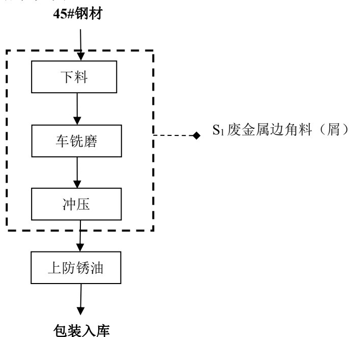
图 1 电机轴生产工艺及产污环节
