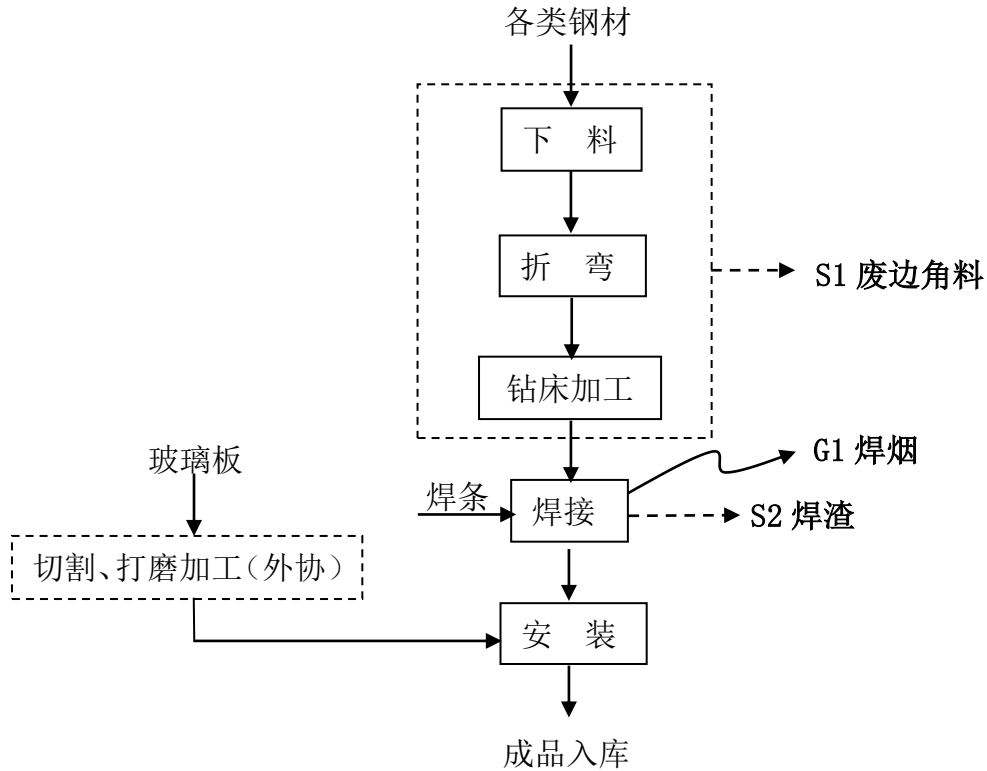
图 1 眼镜展柜厂内生产工艺流程图
