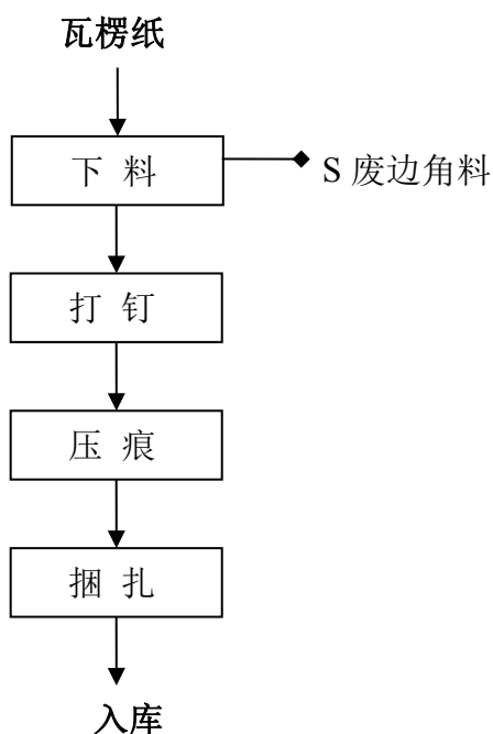
图 1 纸箱生产工艺及产污环节
