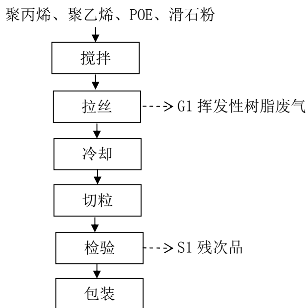
图 2.2-1: PP 改性粒子生产工艺流程及产污环节框图
