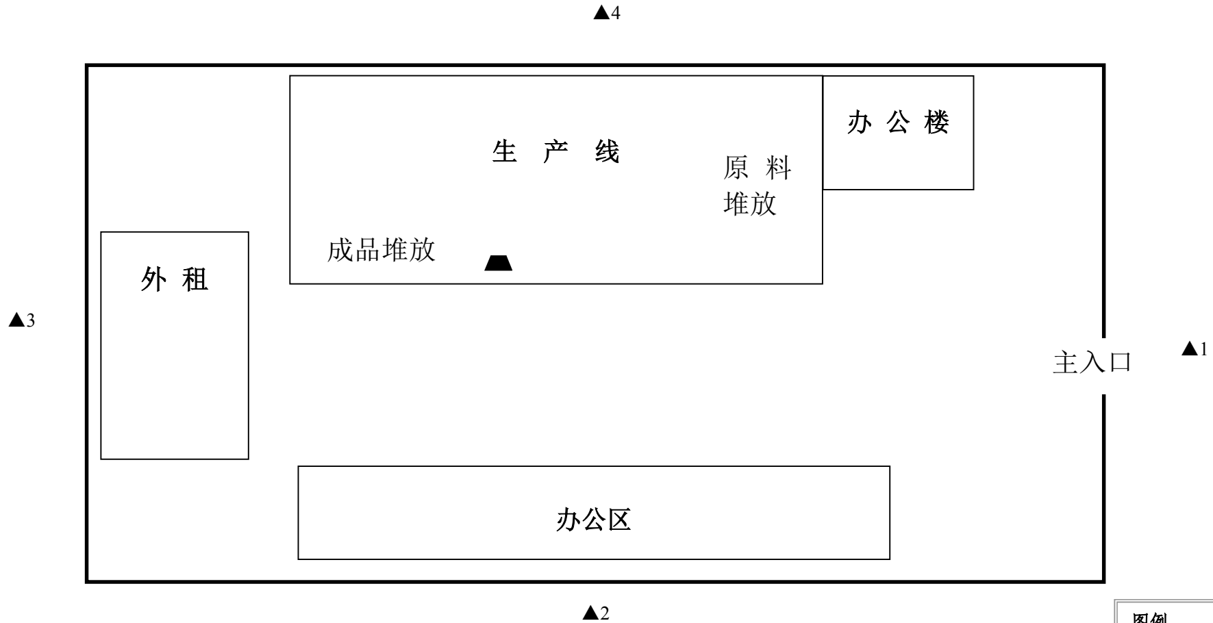
附图3 建设项目全厂平面布置示意图
