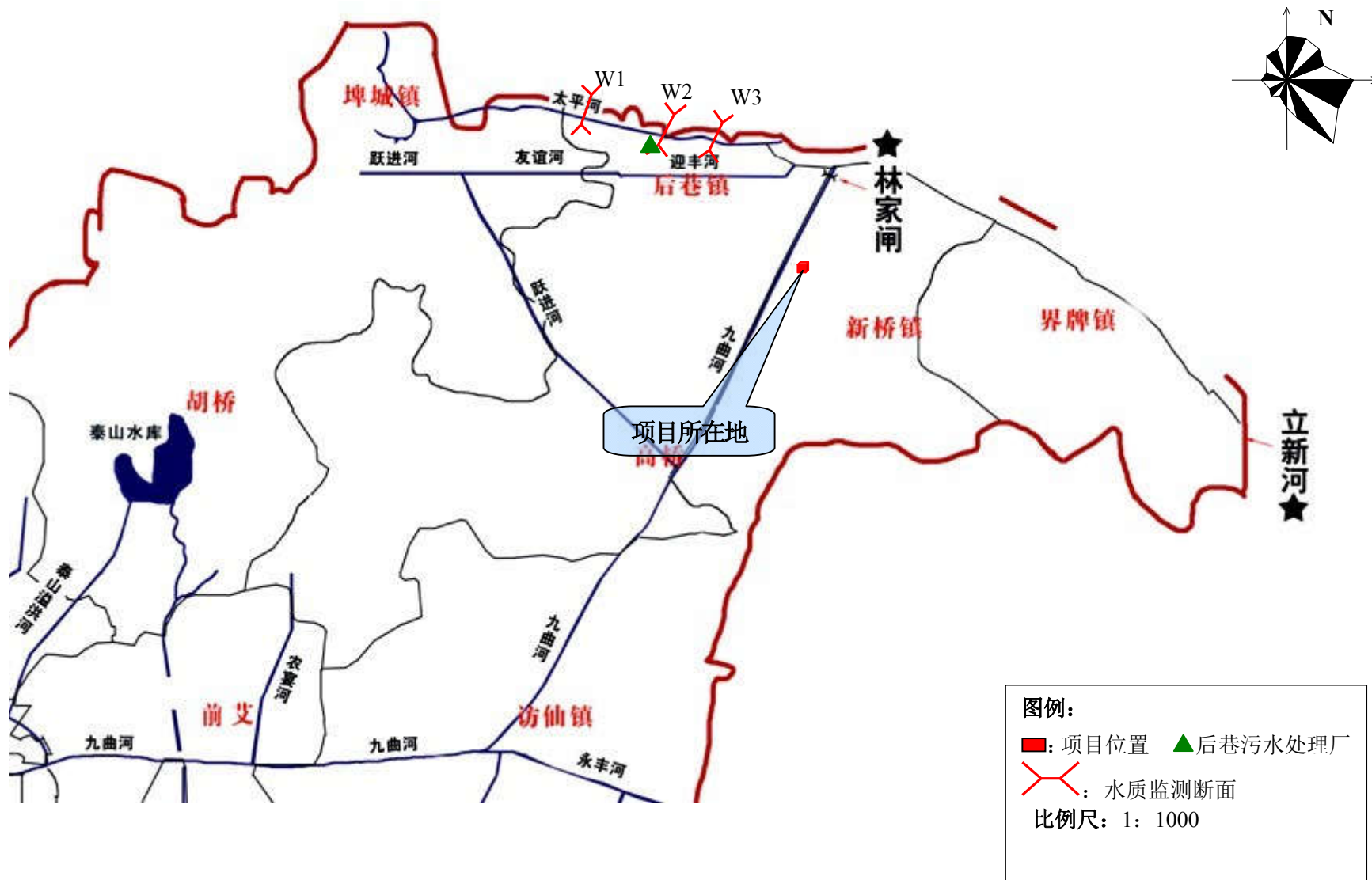
附图 4 本项目所在地区域水系概况图(附水质监测断面)
