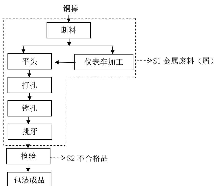
图 2.2-1 接插件螺丝生产工艺流程及产污环节图
