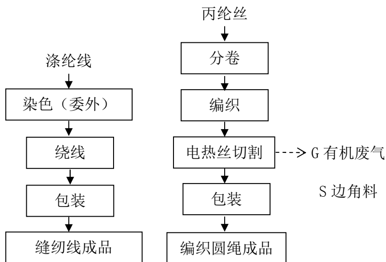
图 2.2.1-1 生产工艺流程框图及主要产污环节图
