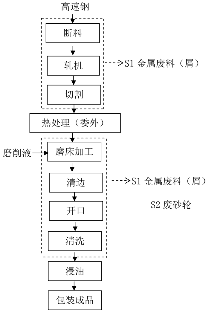
图 2.2-1: 钻头生产工艺流程及产污环节框图
