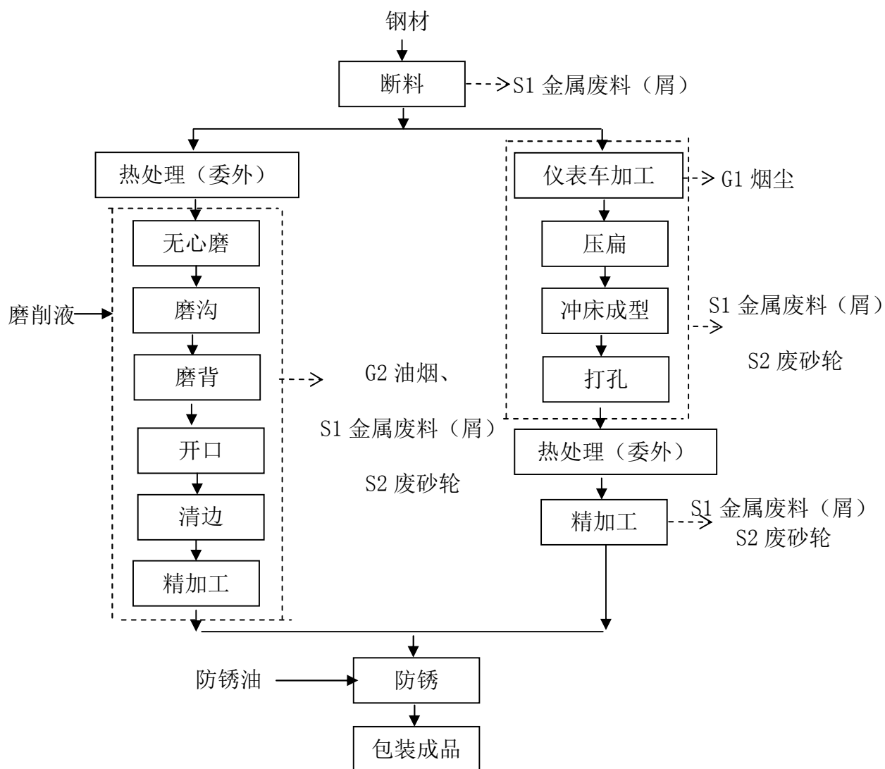
图 2.2-1: 钻头生产工艺流程及产污环节框图
