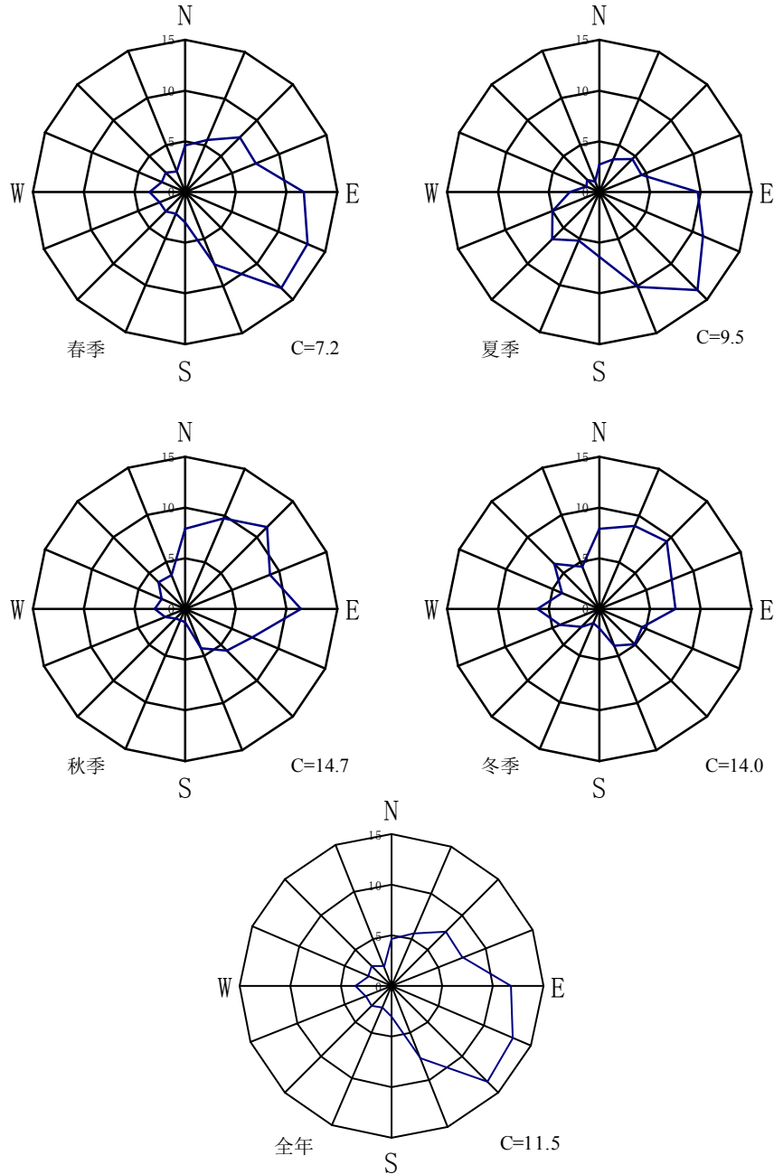
图 4.1-2 丹阳市风向频率玫瑰图
