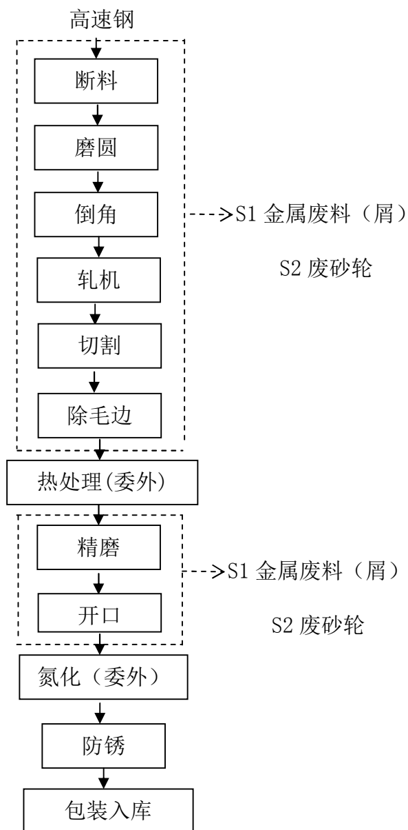
图 2.2-1: 钻头生产工艺流程及产污环节框图
