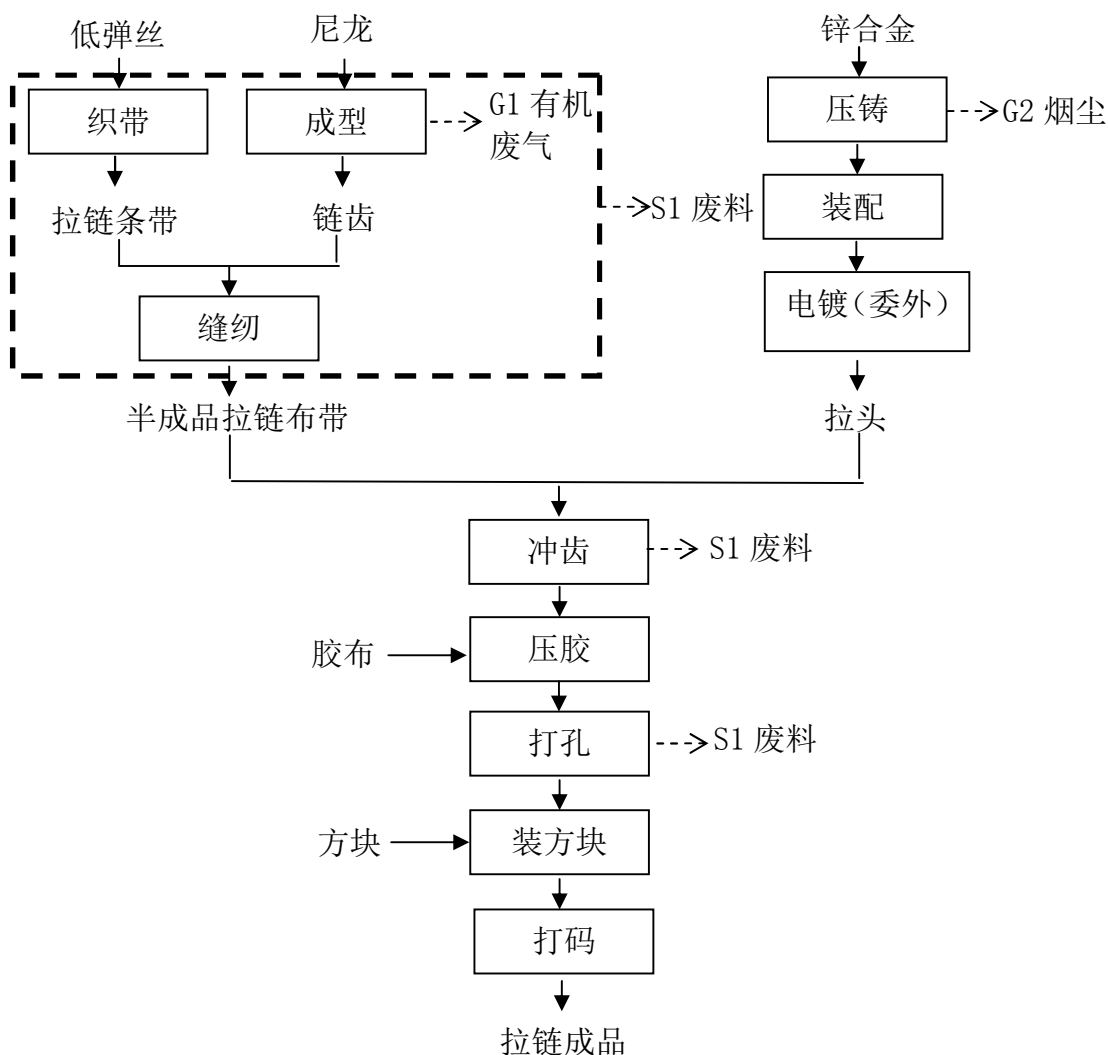
图 2.2.1-1 本项目拉链生产工艺流程框图及主要产污环节图
