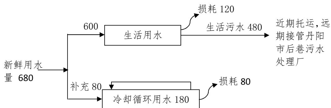
图 2.2-2 本项目用水排水平衡图 (t/a)
