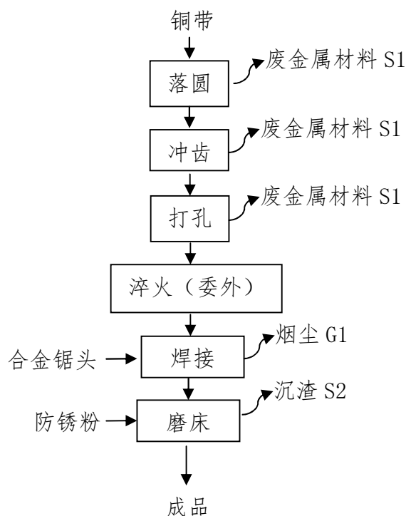
图 2.2-1 合金锯片生产工艺流程及产污环节图
