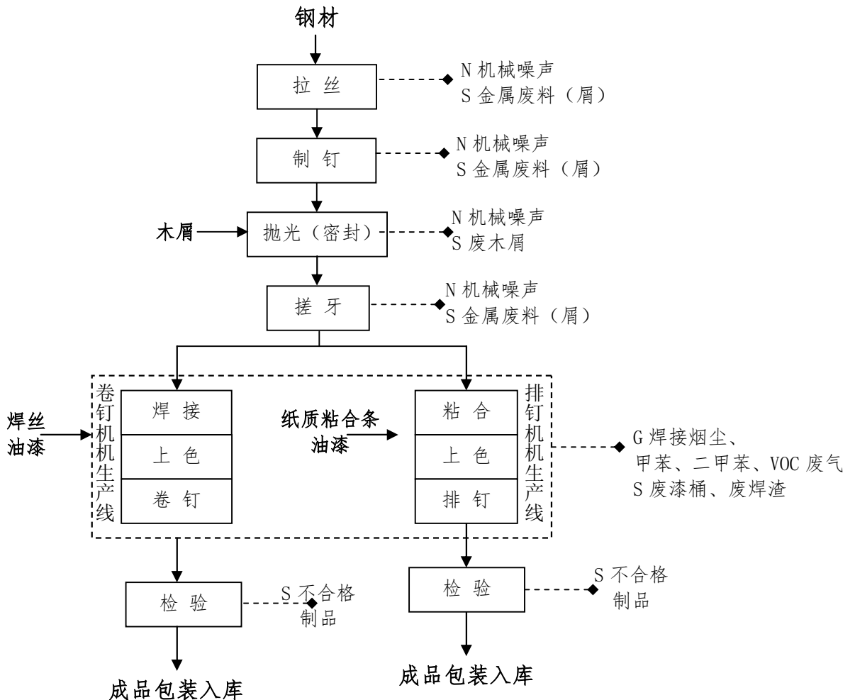
图 2.2-1 本项目五金工具生产工艺流程及产污环节图
