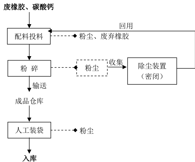
图 2.2-1 项目工艺流程及产污环节框图
