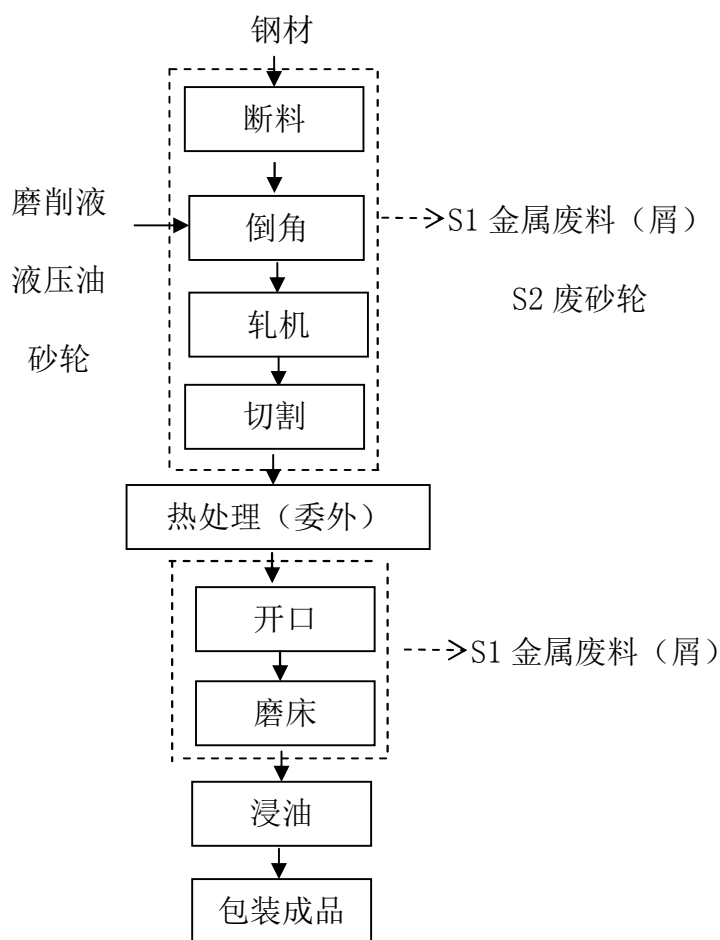
图 2.2-1：钻头生产工艺流程及产污环节框图
