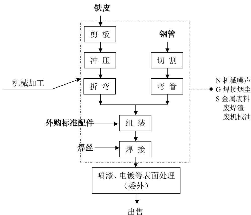
图 2.2-1 本项目生产工艺流程框图及主要产污环节图
