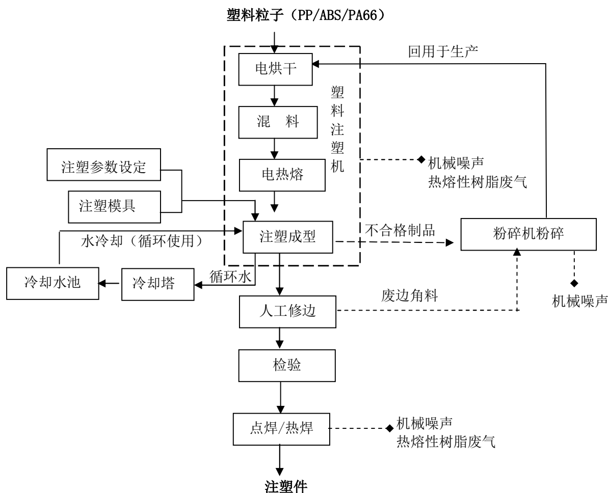
图 2.2-1 塑料件注塑成型工艺流程及产污环节图
