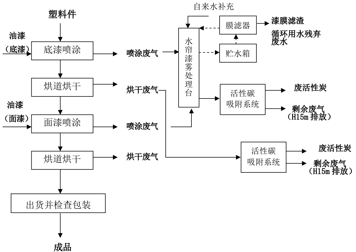
图 2.2-2 塑料件喷涂加工生产工艺流程及主要产污环节图
