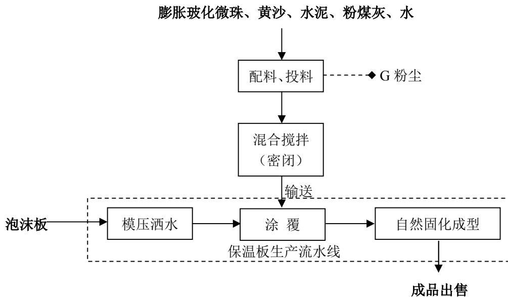
图 2.2-1 项目工艺流程及产污环节框图
