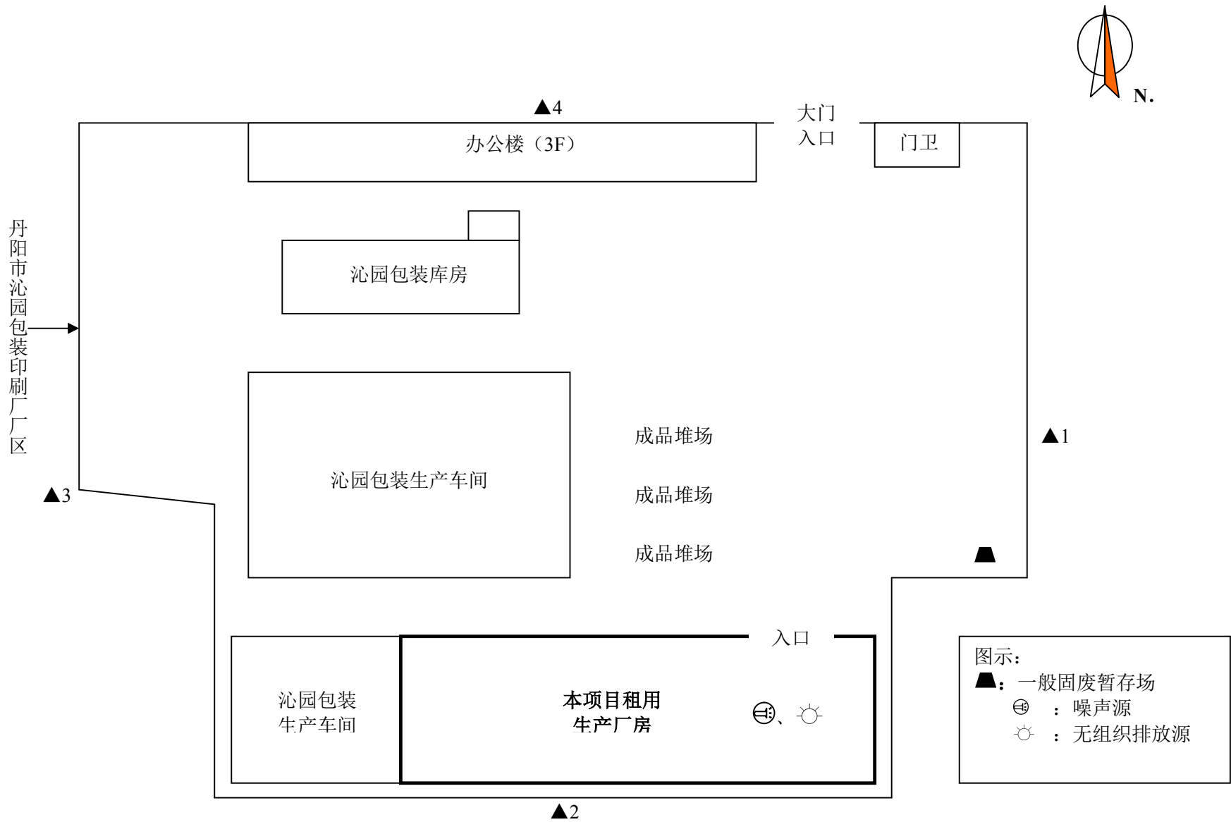
附图2 项目厂区平面布置图 (附噪声监测点)
