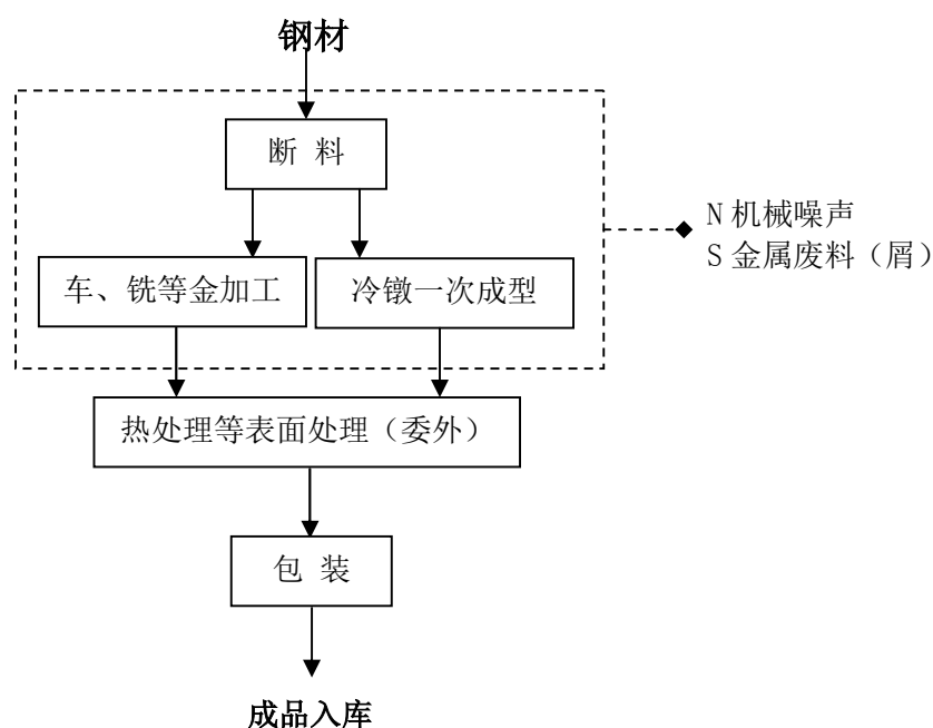
图 2.2-1 本项目五金生产工艺流程及产污环节图
