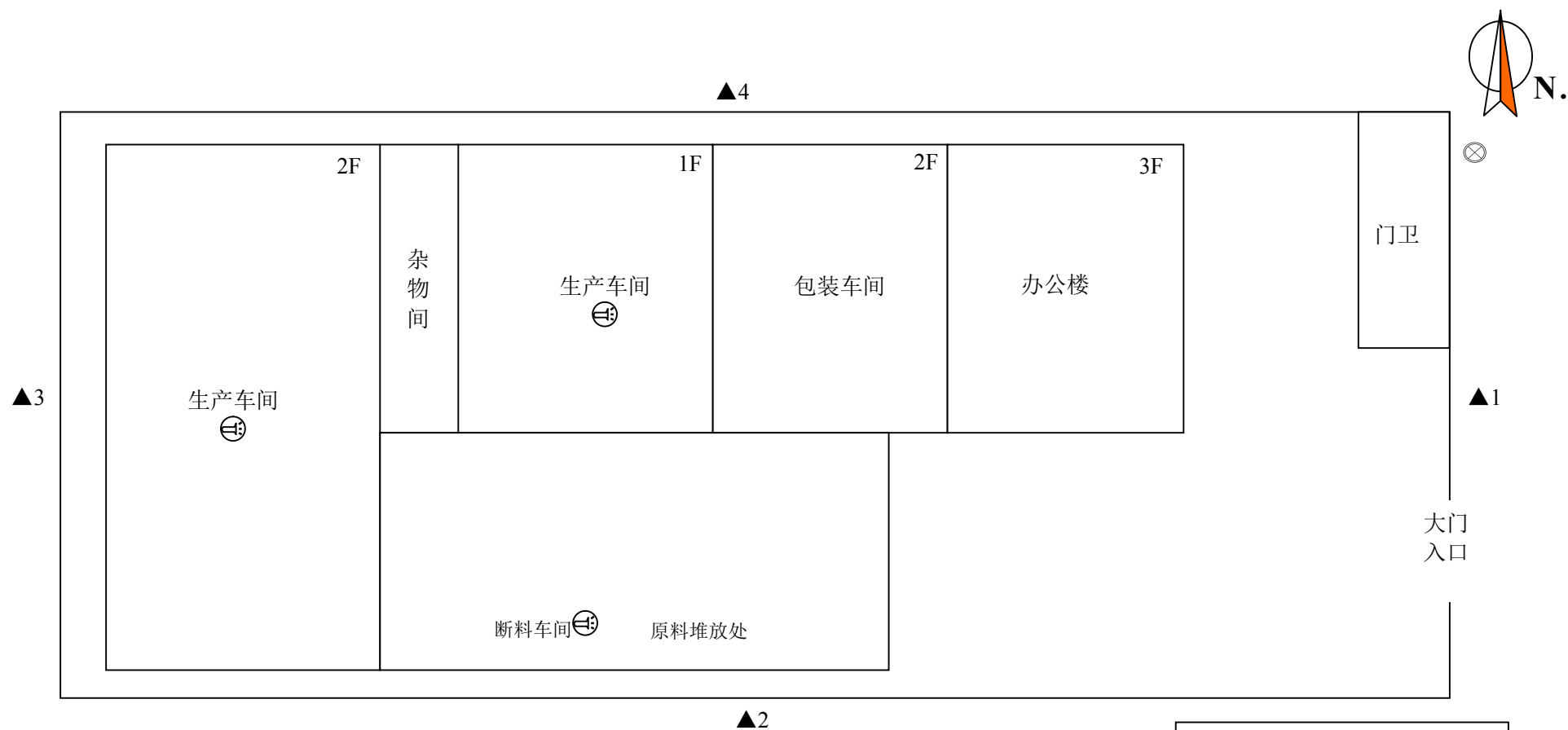
附图2 本项目厂区平面布置图（附噪声监测点）
