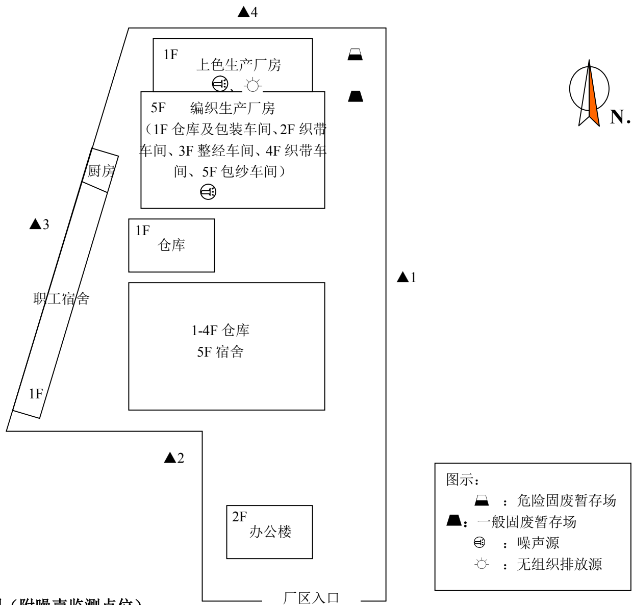
附图2 本项目厂区平面布置图（附噪声监测点位）
