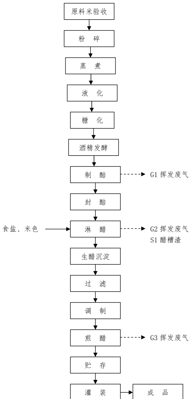
图 2.2-1 项目生产工艺流程及产污环节框图
