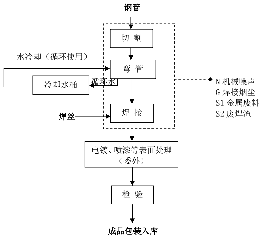
图 2.2-1 本项目汽车配件生产工艺流程及产污环节图
