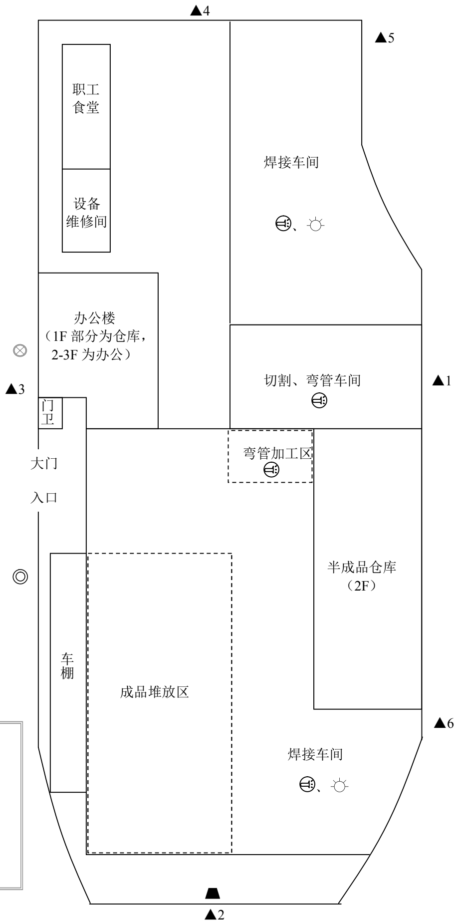
附图 2 本项目厂区平面布置图(附噪声监测点位)
