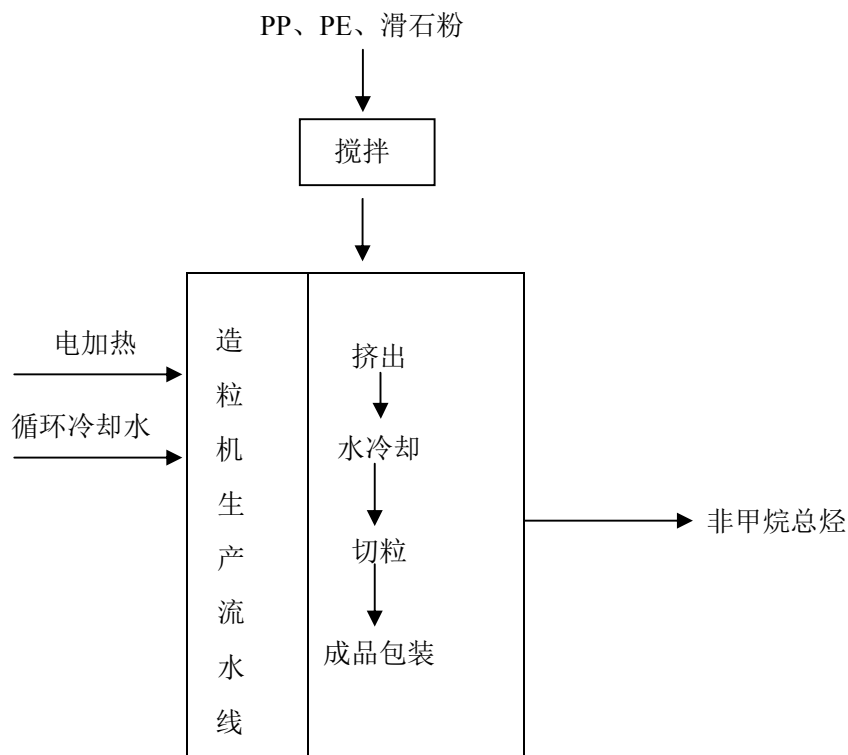
图 1 生产工艺及产污环节图
